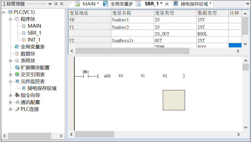
图4-11 子程序 SBR_1 的编写过程
