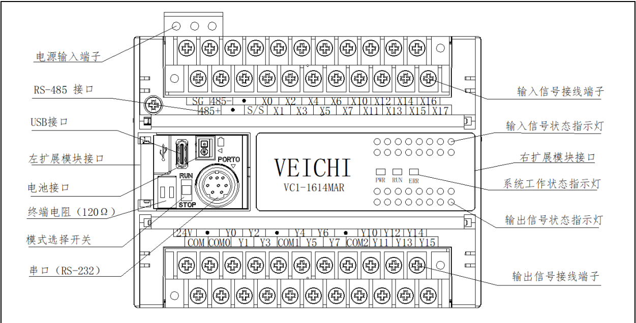
图1-1 VC1 系列主模块外形结构
