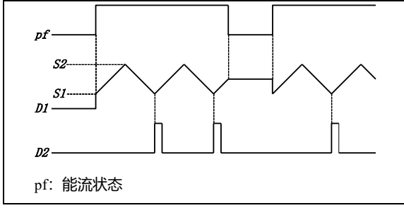
三角波指令执行过程分解如下图（S3=5）：
