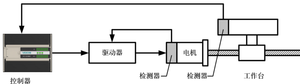
图11-4 闭环控制系统简图
