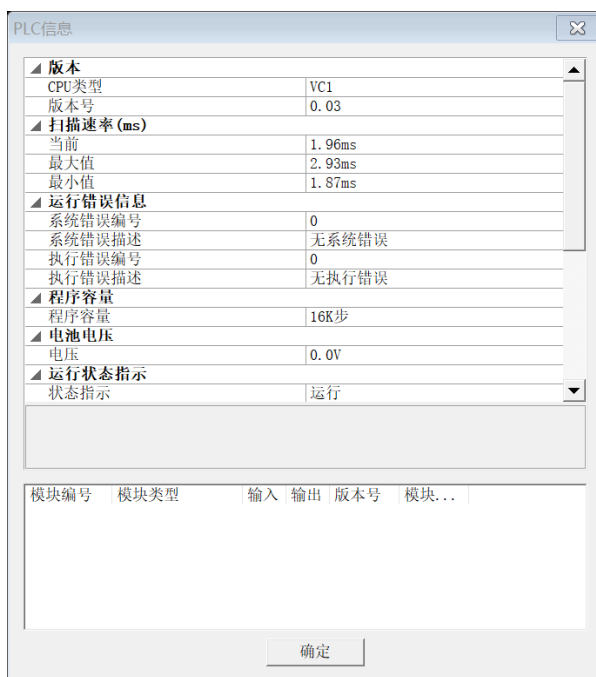
图2-17 PLC 当前运行信息
