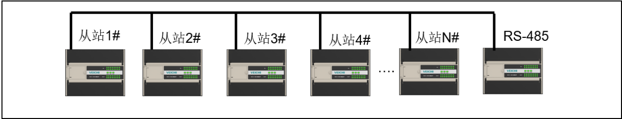
图10-7 N:N 单层网络
