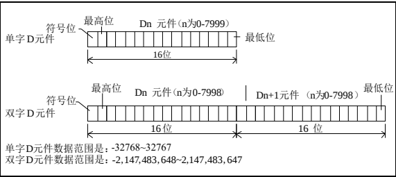
图3-5 D 或 R 元件
