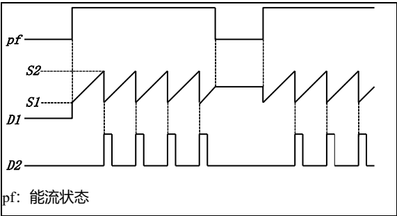
锯齿波指令执行过程分解如下图（S3=5）：
