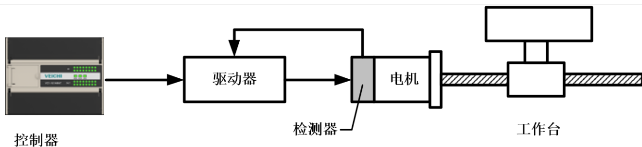
图11-5 半闭环控制系统简图
