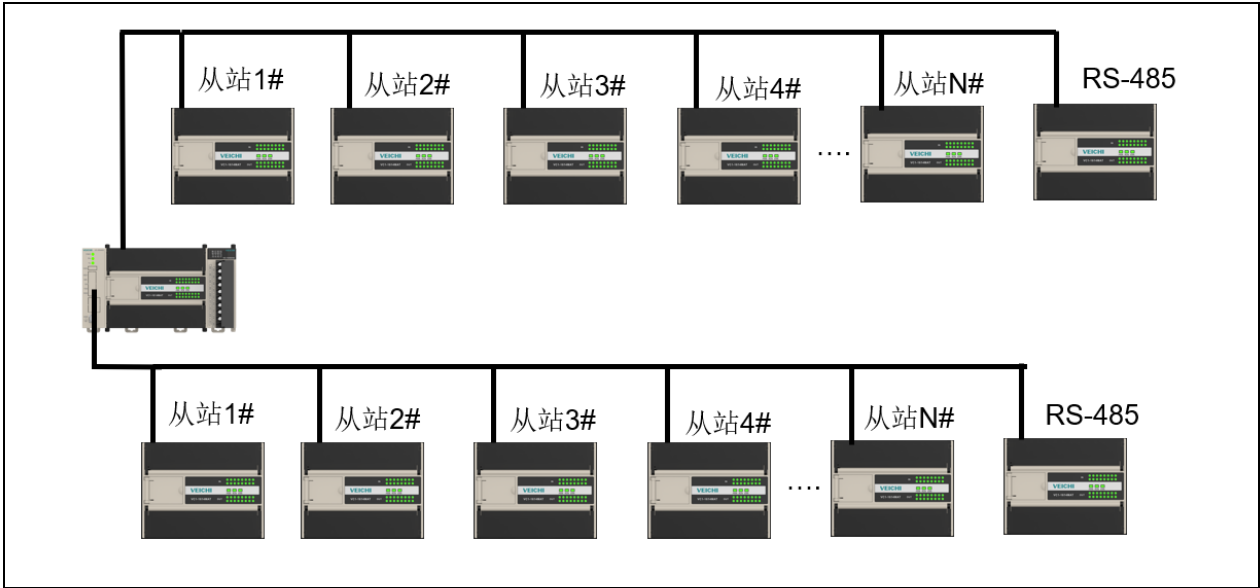
图10-8 N:N 多层网络
