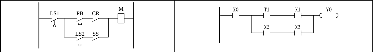
图4-1 电气控制图和梯形图的等效关系
