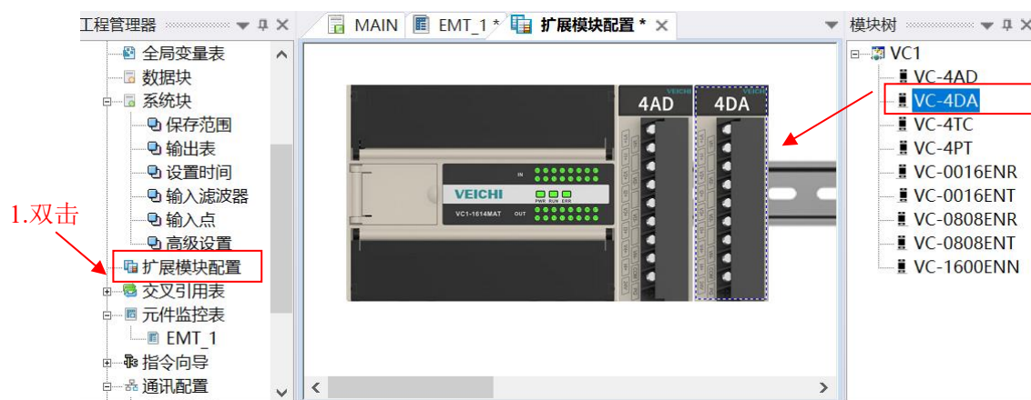
图2-10 配置特殊模块
