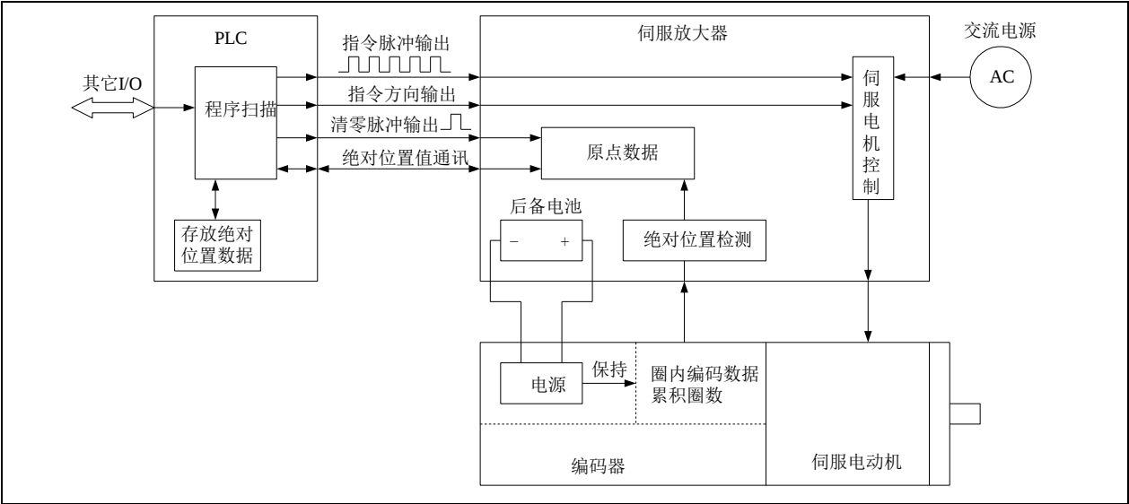
图11-1 绝对位置系统功能图
