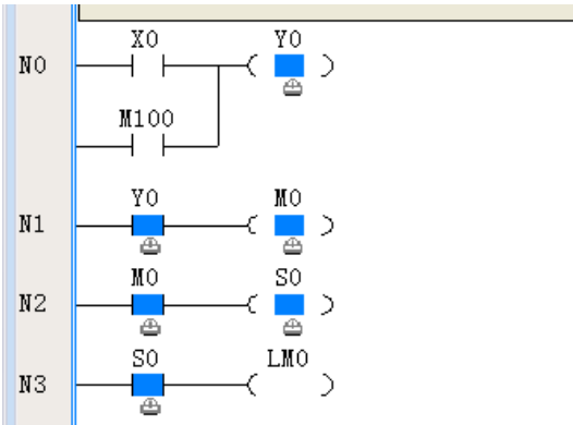
图2-21 被强制软元件的锁标记
