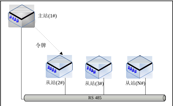
图10-2 主站向2#从站发放令牌
