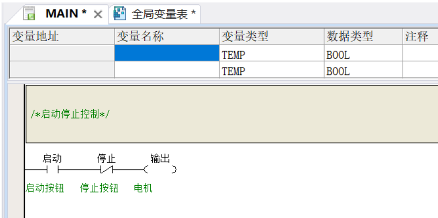
图4-10 显示元件注释时的梯形图程序
