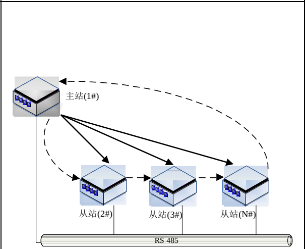
图10-6 令牌的发放与流动顺序
