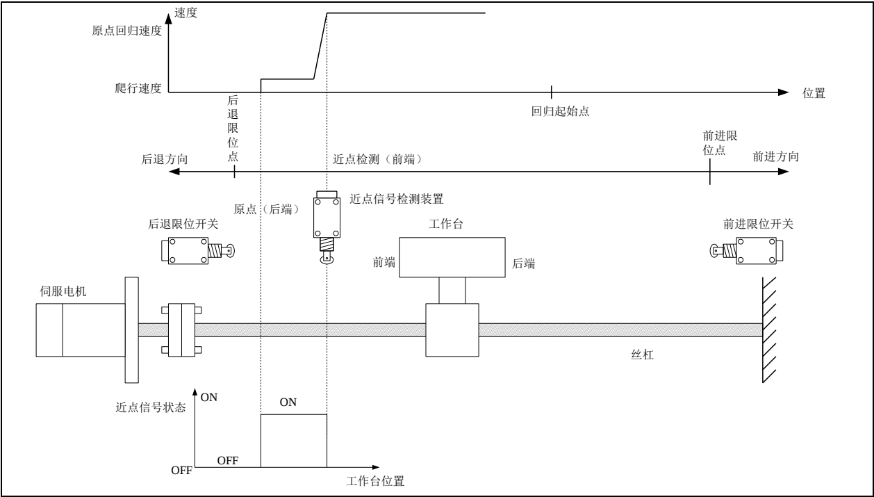
图11-2 绝对位置系统机械示例简图
